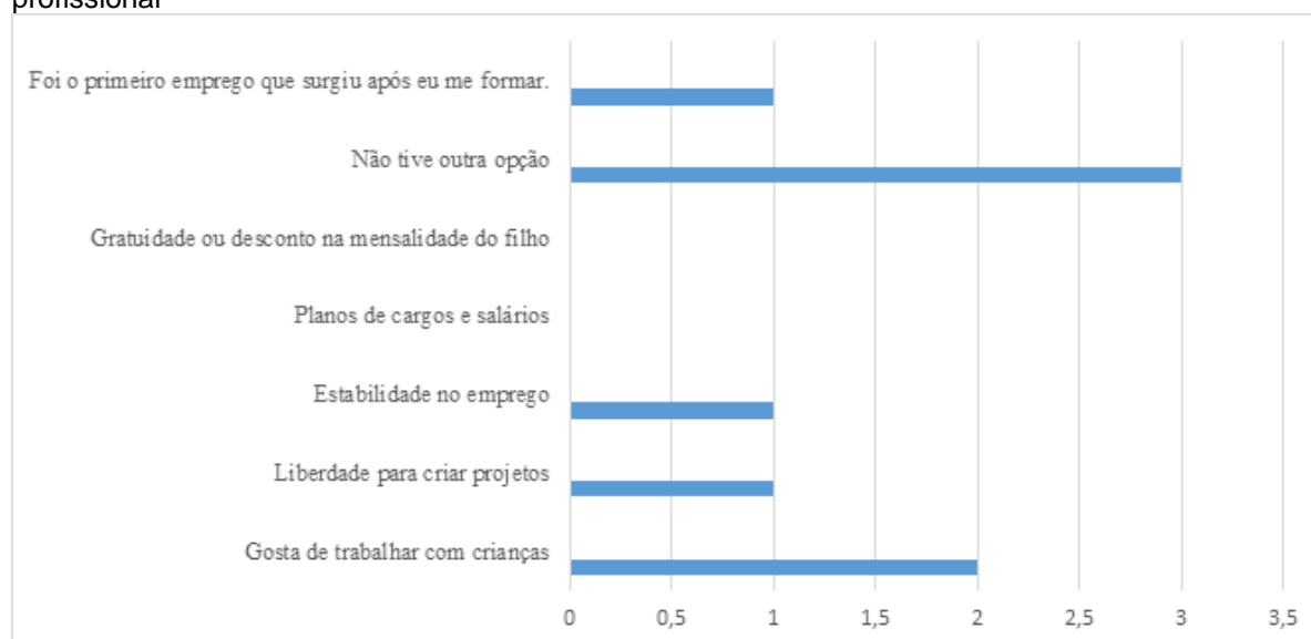
Gráfico 1 - Motivação profissional
